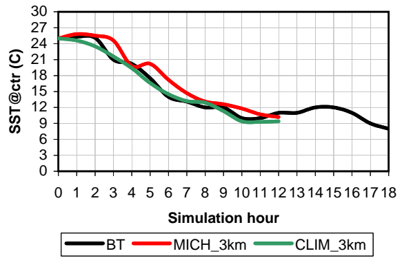
SST @ctr (3km)
