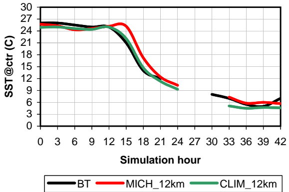
SST @ctr (12km)
